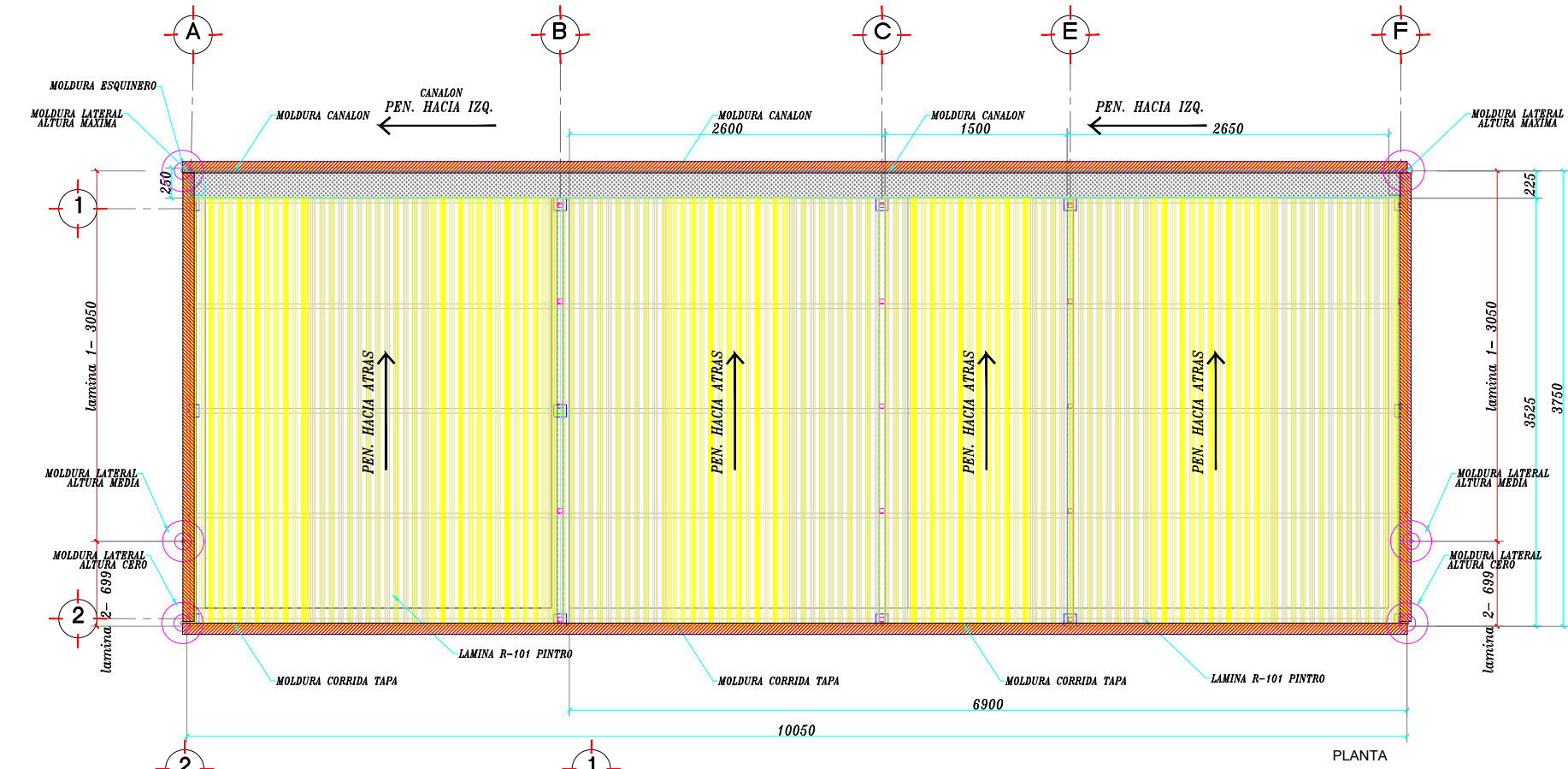
VISTA TRABE DE PTR 2" Y BASTIDOR 1-1'
